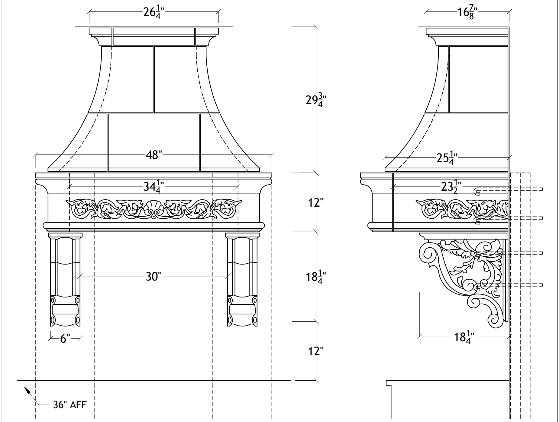
30" Mini Le Petite Range Hood for 9' ceiling
