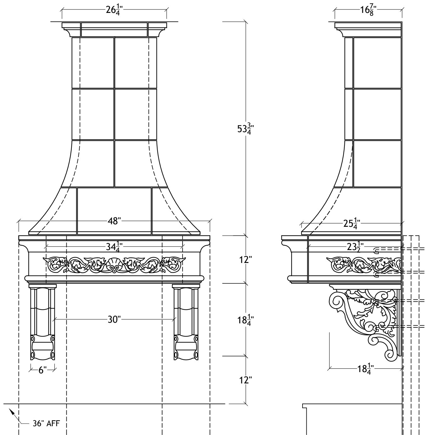
30" Mini Le Petite Range Hood for 11' ceiling
