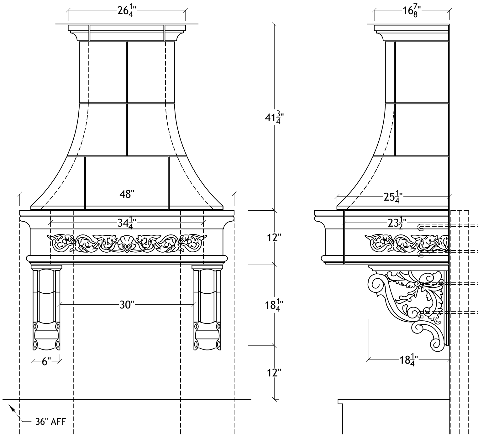
30" Mini Le Petite Range Hood for 10' ceiling
